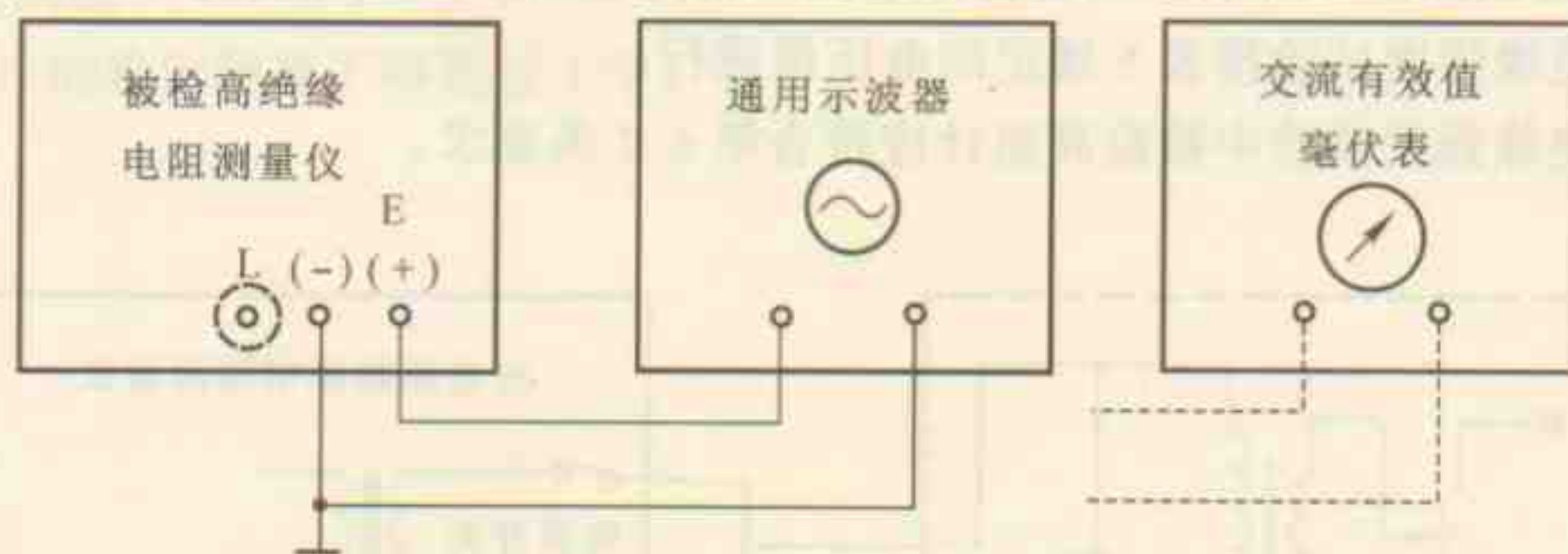
图 2 端钮电压纹波分量测量接线图
