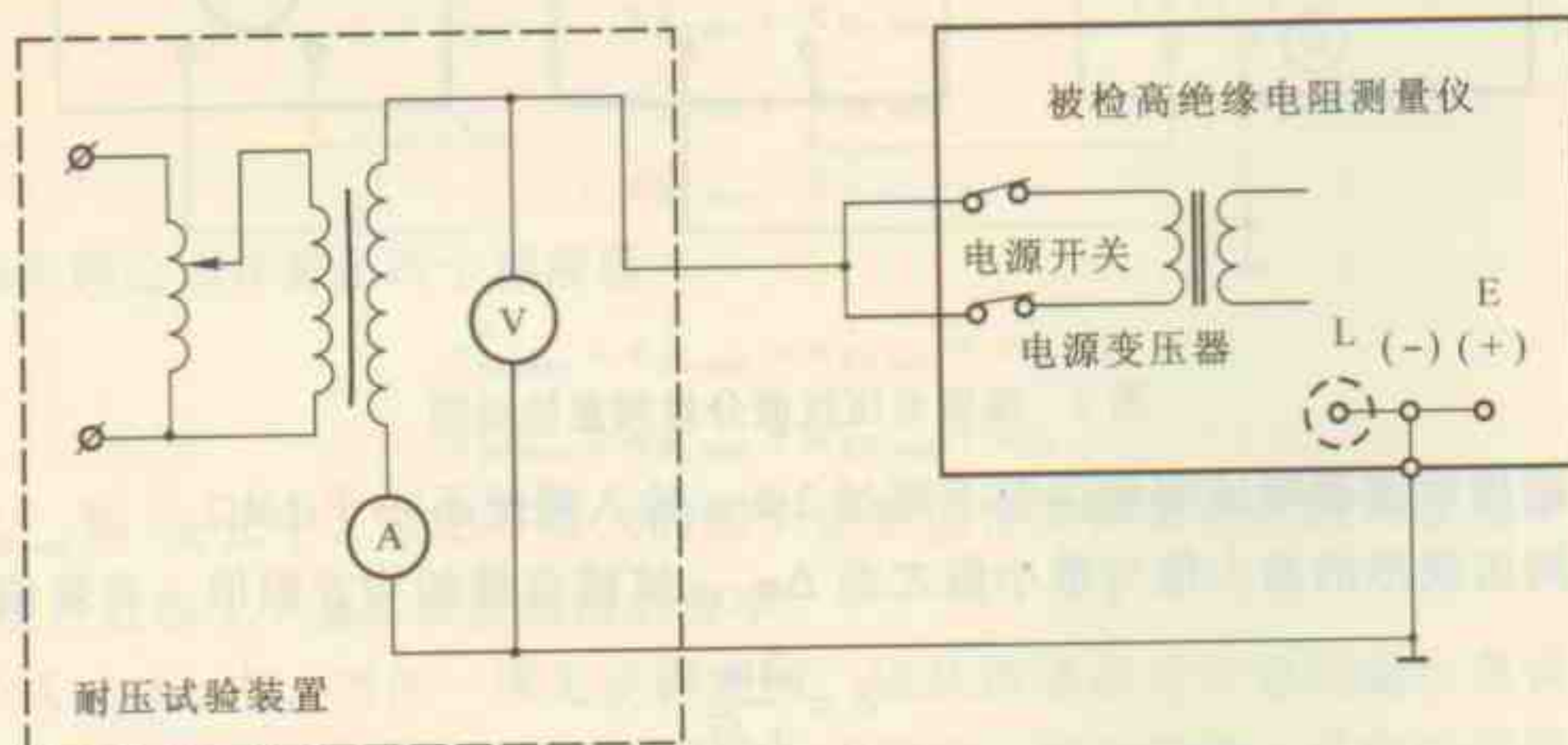
图4 绝缘强度试验接线图
